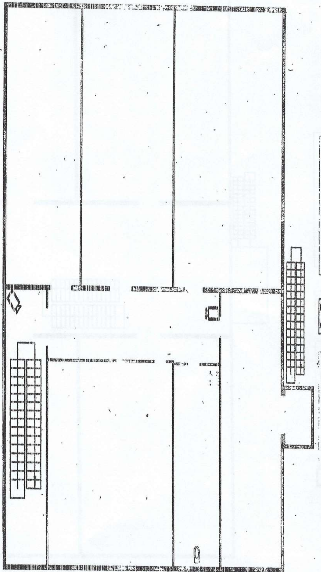
Принципиальная схема устройства видеонаблюдения в ГКС(К)ОУ "Специальная (коррекционная) общеобразовательная школа-интернат №10 Ул. Вийде" пгт. Б 2 этаж
